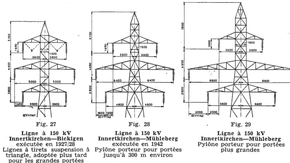
Fig. 27, 28 et 29 Dispositions des câbles conducteurs
