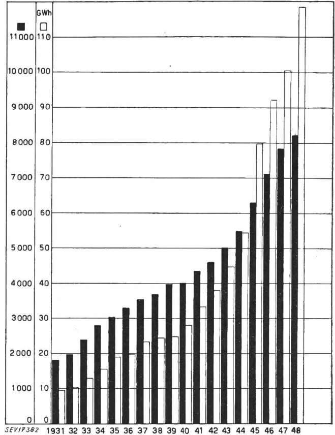
SEV17382 Fig. 2 Fourneaux de cuisines professionnelles En noir: Nombre de fourneaux; en blanc: Consommation
