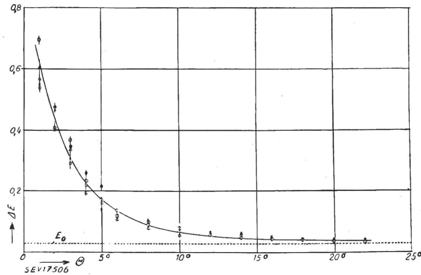
Fig. 4 Nötige Erhöhung der Beleuchtungsstärke \Delta E zur Sichtbarmachung des Objektes bei verschiedenem Winkelabstand \theta der blendenden Lichtquelle
