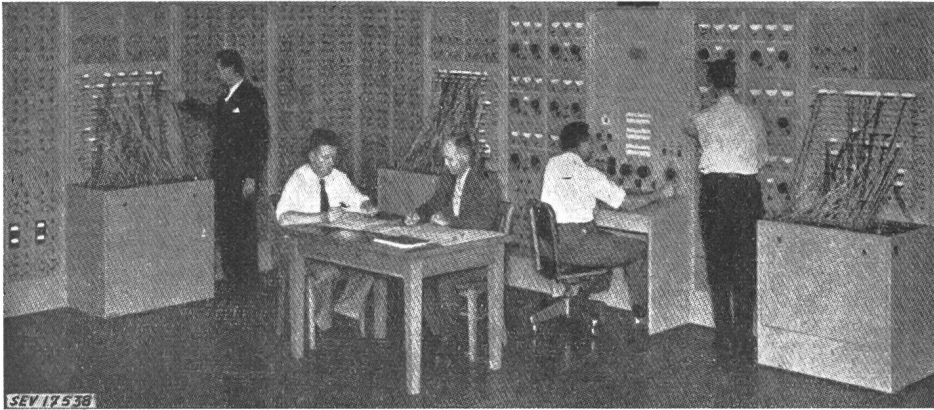
Fig. 5 Wechselstromnetzmodell der Denver Federal Center
