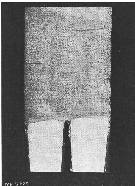
Fig. 4 Schliffbild einer 6-mm-Draht-Schweissung (geätzt, 5fache Vergrößerung)
