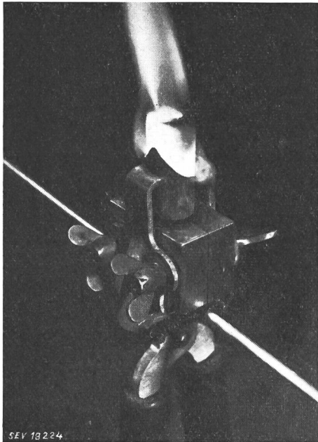
Fig. 3 Schweiss-Patrone während des Abbrennens
