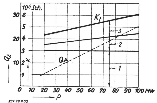
Fig. 3 Kosten eines Wasserkraftwerkes mit Jahresspeicherung und reiner Winterproduktion Q_A Ausbauleistung; K Jahreskosten in Millionen Schilling; K_t totale Jahreskosten; P installierte Leistung; Aufteilung der Jahreskosten: 1 Speicher, 2 Stollen, 3 Rohrleitung und Maschinenhaus
