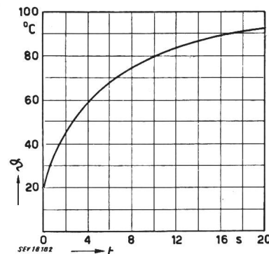
Fig. 12 Verlauf der Temperatur \theta in der Leimnaht als Funktion der Zeit t
