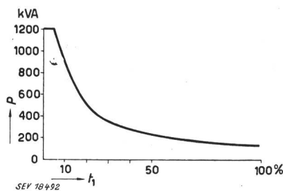
Fig. 6 Schallleistung zweier Ignitrons in Gegentaktschaltung in Funktion der Einschaltdauer Grenzleistung = 1200 kVA, 380 V t 1 Einschaltdauer (Integrationszeit = 8 s); P Leistung
