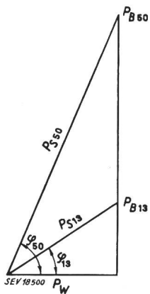
Fig. 13 Leistung und Leistungsfaktor einer 1-Phasenmaschine 50 Hz und einer 3-Phasenmaschine 13 Hz bei gleicher Nutzleistung P_{B\ 50} = 230\text{ kVA}; P_{B\ 13} = 65\text{ kVA}; P_{S\ 50} = 250\text{ kVA}; P_{S\ 13} = 118\text{ kVA}; \cos \varphi_{50} = 0,4; \cos \varphi_{13} = 0,85; P_W = 100\text{ kW}
