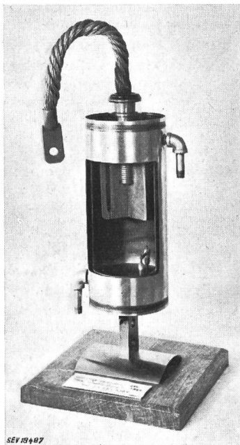
Fig. 1 Ignitron Schältröhre Maximale Schaltleistung 1200 kVA
