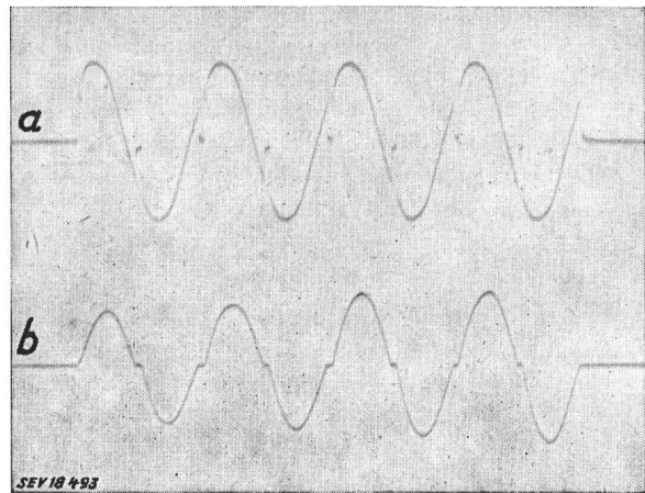
Fig. 7 Oszillogramm des Schweißstromes und der Spannung am Transformator beim Punktschweissen mit einer Schweisszeit von 0,08 s a Spannung; b Strom
