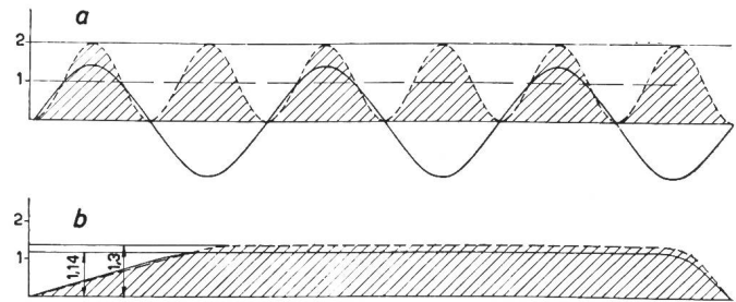
Fig. 14 Vergleich des zeitlichen Verlaufs des Schweißstromes I und der Wärmeleistung I^2R bei gleicher Schweissenergie (Oberwellen vernachlässigt) a 50-Hz-Schweissmaschine; b Frequenzwandler-Schweissmaschine; R Widerstand an der Stromübergangsstelle — Schweißstrom - - - - - Wärmeleistung I^2R
