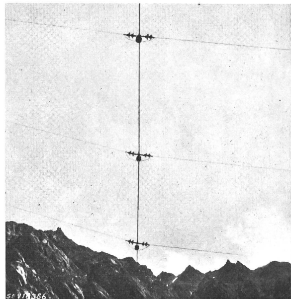
Fig. 6 Queraufhängung
