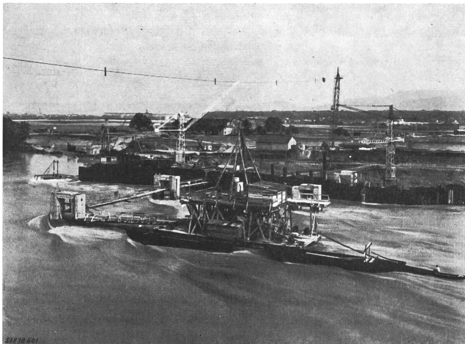
Fig. 1 Blick vom rechten Rheinufer gegen die Baugrube des Trennpfeilers Links im Bild der ehemalige Flugplatz Sternenfeld (Sommer 1951)
