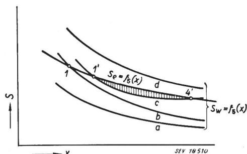
Fig. 3 Vergleich der s_w - und s_e -Kurven Erläuterungen im Text
