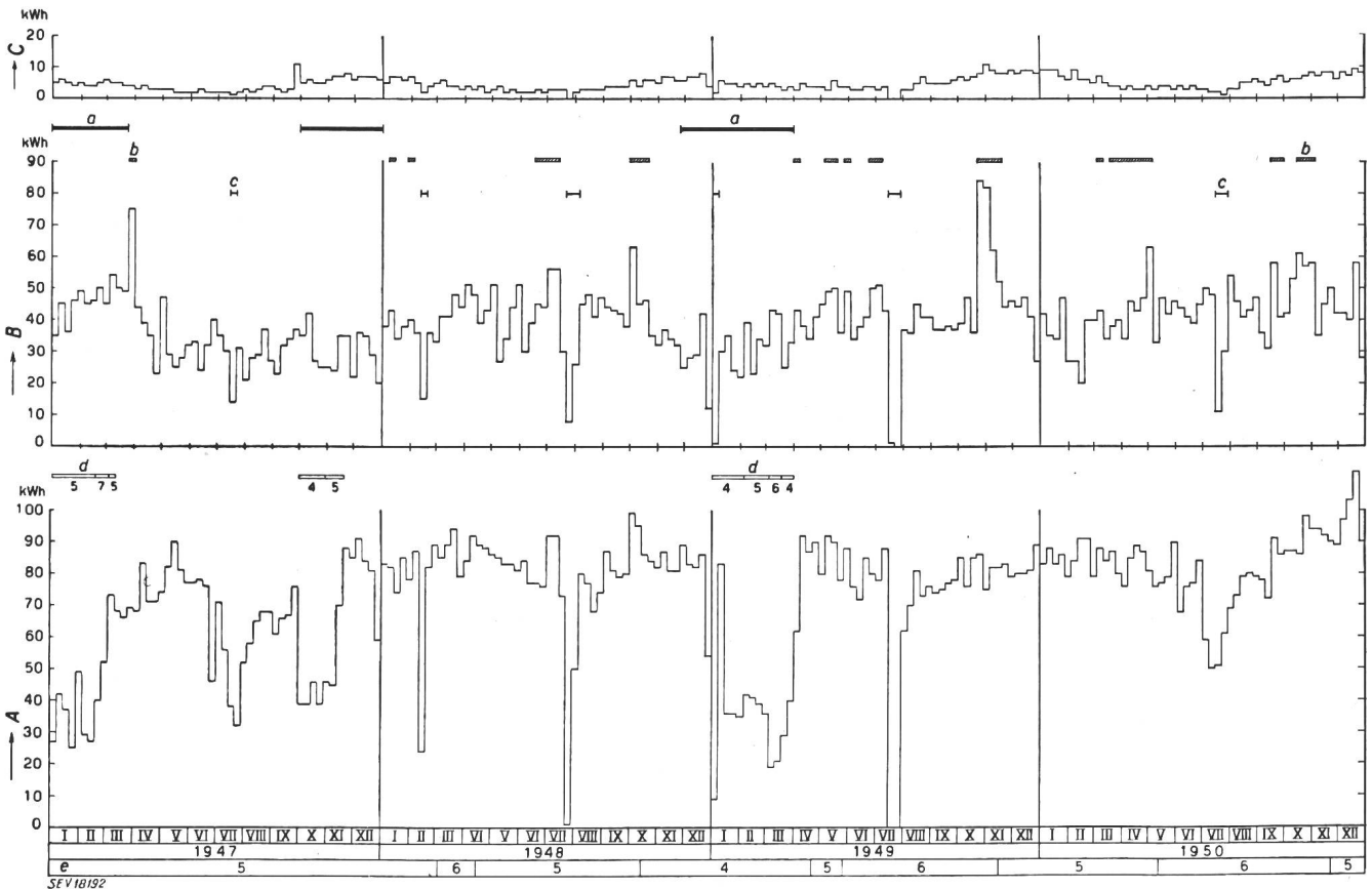
Fig. 1 Consommation hebdomadaire d'électricité dans une maison familiale de 7 pièces, 1947...1950 A Applications thermiques TB (nuit) b Chauffage d'appoint en service B Applications thermiques TH (jour) c Vacances C Eclairage d Interdiction de la préparation d'eau chaude, en jours par semaine a Restrictions du chauffage des locaux e Nombres de personnes du ménage
