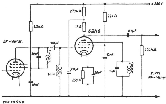
Fig. 10 FM-Demodulationsstufe mit der Röhre 6BN 6
