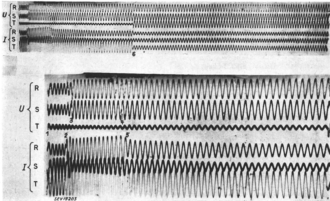
Fig. 3 Oszillogramm der Störung vom 15. September 1950 Aufgenommen in Gösgen auf der Parallelleitung B der Fig. 2 oben: ganzer Oszillogrammstreifen verkleinert unten: Anfang des Streifens vergrössert
