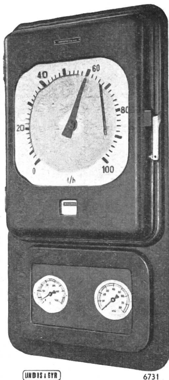
Fig. 4 Mitteldruck-Ringwaage für Dampfmengenmessung und -zählung mit Kreisblatt-Registrierung sowie Druck- und Temperatur-Korrekturvorrichtung
