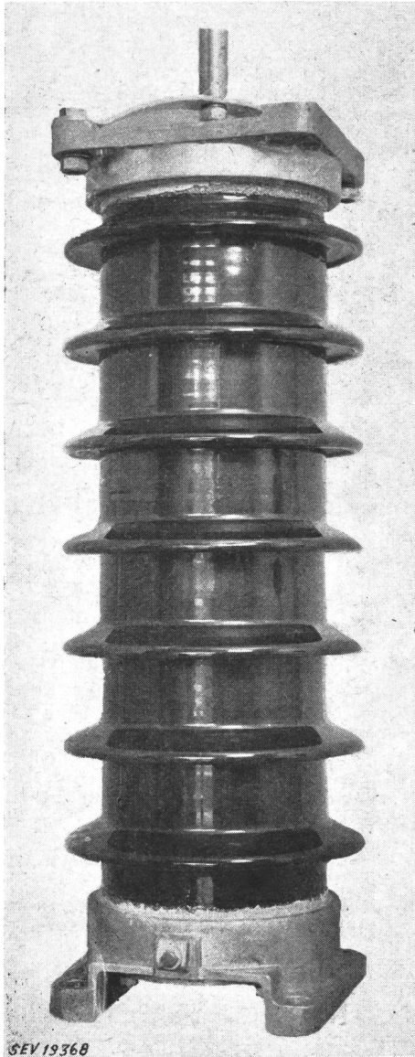
Fig. 1 Überspannungsableiter Typ BHF
