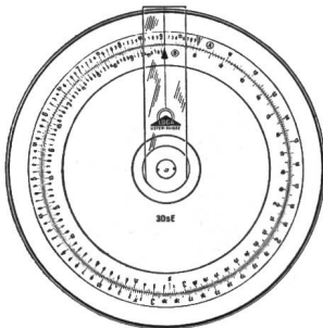
Fig. 2 Cos \varphi - Rechenscheibe Vorderseite
