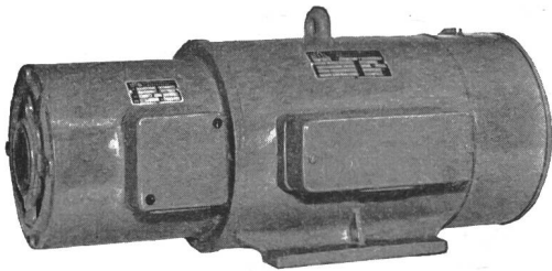
Fig. 3 Asynchron-Frequenzumformer (50 auf 150/250 Hz) mit angebautem Antriebmotor
