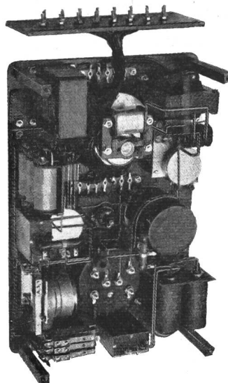
Fig. 3 Spannungs-Programmregler Innenansicht
