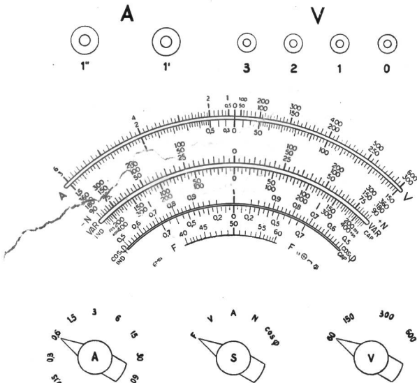
Fig. 2 Skala des Vancos-Meters
