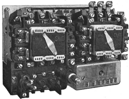
Fig. 1 Stern-Dreieck-Schütz 40 A
