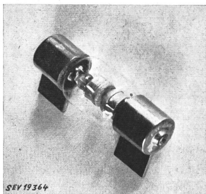
Fig. 1 Gasgefüllter Überspannungsableiter
