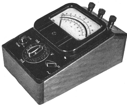
Fig. 1 Tragbares Vielfachmessgerät
