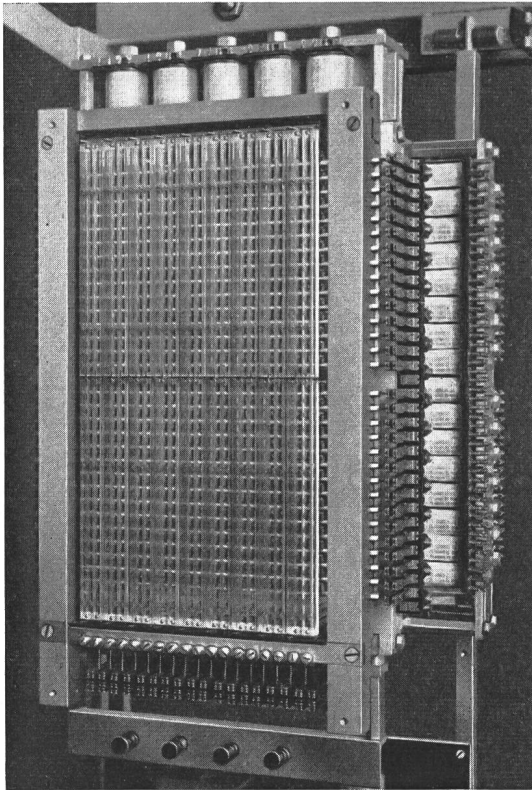
Fig. 1 Kreuzwähler für Telephonautomat
