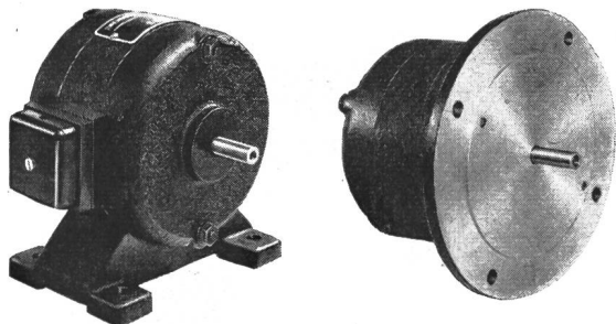
Fig. 2 Tachometer-Ferngeber
