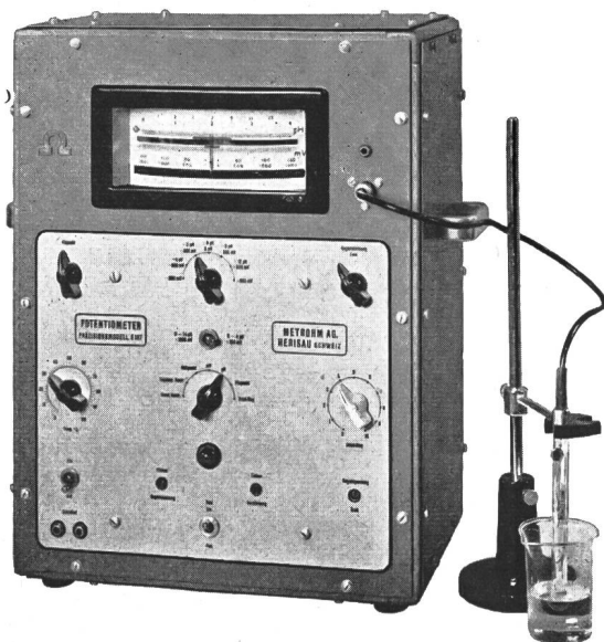
Fig. 2 Präzisionspotentiometer
