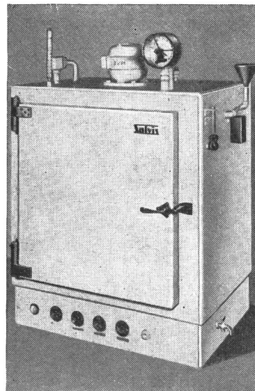
Fig. 1 Elektrischer Klimaschrank mit automatischer Luftkonditionierung und kombiniertem Heiz- und Kühlsystem
