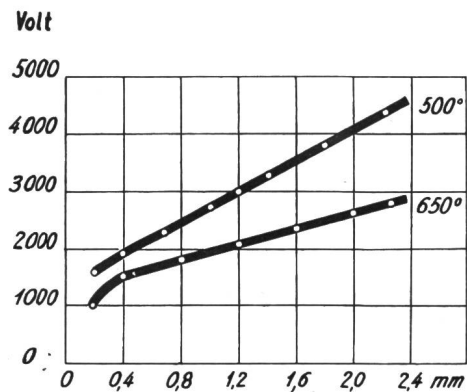
Fig. 6 Durchschlagspannung der keramischen Einbettmasse als Funktion der Schichtdicke und der Temperatur
