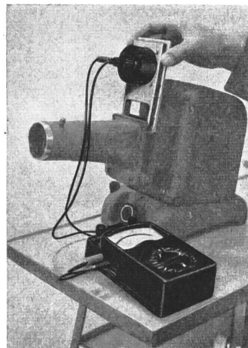
Fig. 4 Multimeter mit Projektionseinheit
