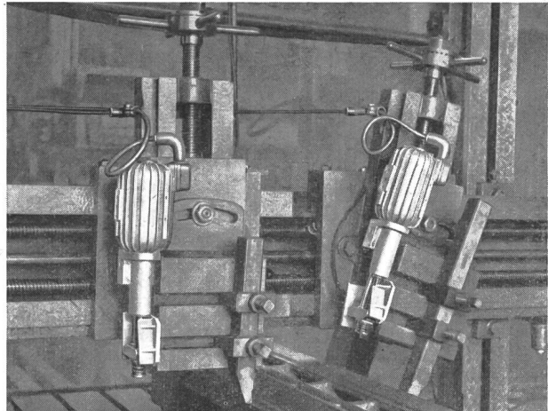
Fig. 1 Querbalken einer Tischhobelmaschine, ausgerüstet mit zwei elektrischen Stahlabhebern ES 1
