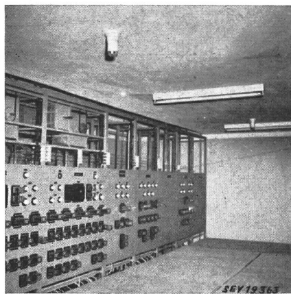
Fig. 2 Ionisations-Feuermelder in der Schaltanlage eines unterirdischen Kraftwerkes
