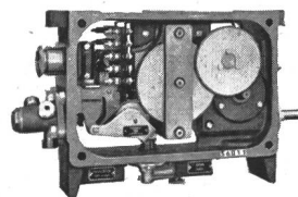
Fig. 3 Oerlikon-Sicherheitsapparat
