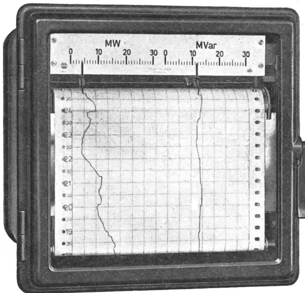
Fig. 2 Quadratisches Registrierinstrument zum Einbau Frontrahmen 240 × 240 mm
