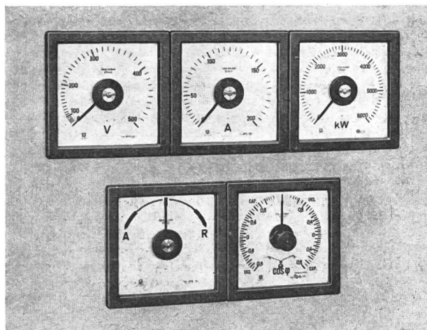
Fig. 1 Schalttafel-Einbau-Instrumente Frontrahmen 110 × 110 mm; Skalenlänge rund 160 mm
