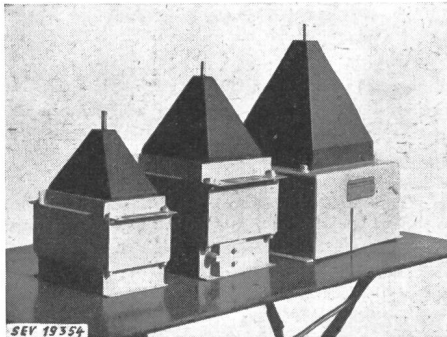
Fig. 1 Kunstharz-Trockenspannungswandler 10, 20, 30 kV
