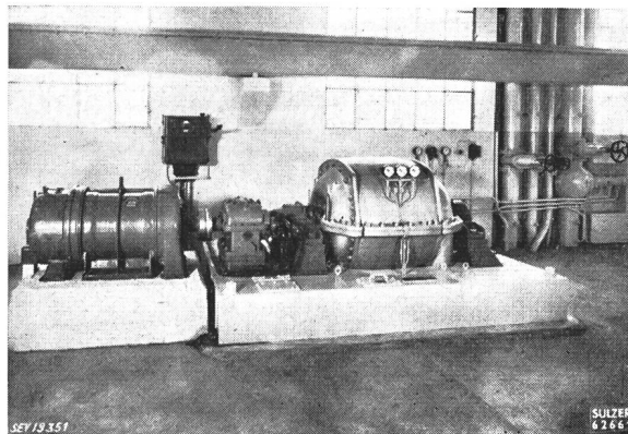
Fig. 1 Mehrstufiges Sulzer-Vakuumgebläse in einer schweizerischen Papierfabrik. Spezialausführung mit grosser, geschweisster Grundplatte, die gleichzeitig als Ölreservoir dient
