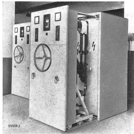
Fig. 2 Schaltzelle in gekapselter Ausführung
