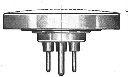
Fig. 2 Darstellung der Durchbiegung f einer elektrischen Kochplatte
