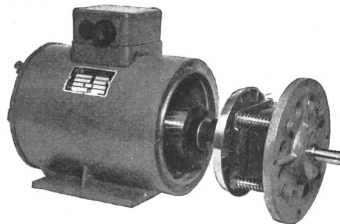
Fig. 2 Stopmotor, geöffnet
