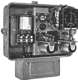
Fig. 2 Ölfeuerungsautomat
