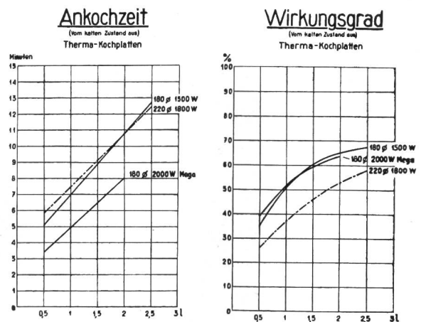
Fig. 2 Ankochzeit und Wirkungsgrad der Megatherma-Platte 18 cm \phi , 2000 W, im Vergleich zu den gewöhnlichen Schnellkochplatten
