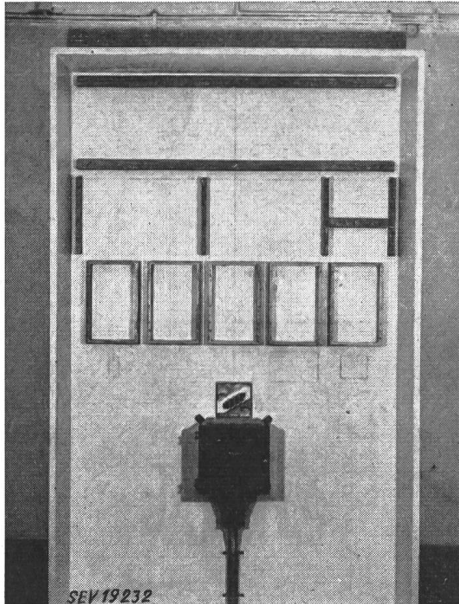
Fig. 20 Début du montage de l'installation de la fig. 17
