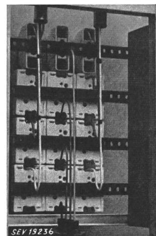
Fig. 24 Ligne conduite derrière des socles de coupe-circuit, verticalement et distancée latéralement
