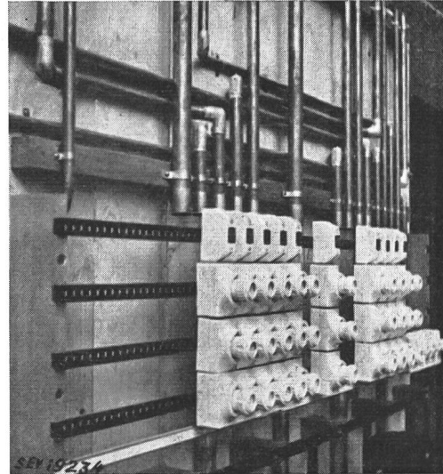
Fig. 22 Modèle d'appareillage de distribution et de protection, avec lignes sur deux plans différents Vue latérale
