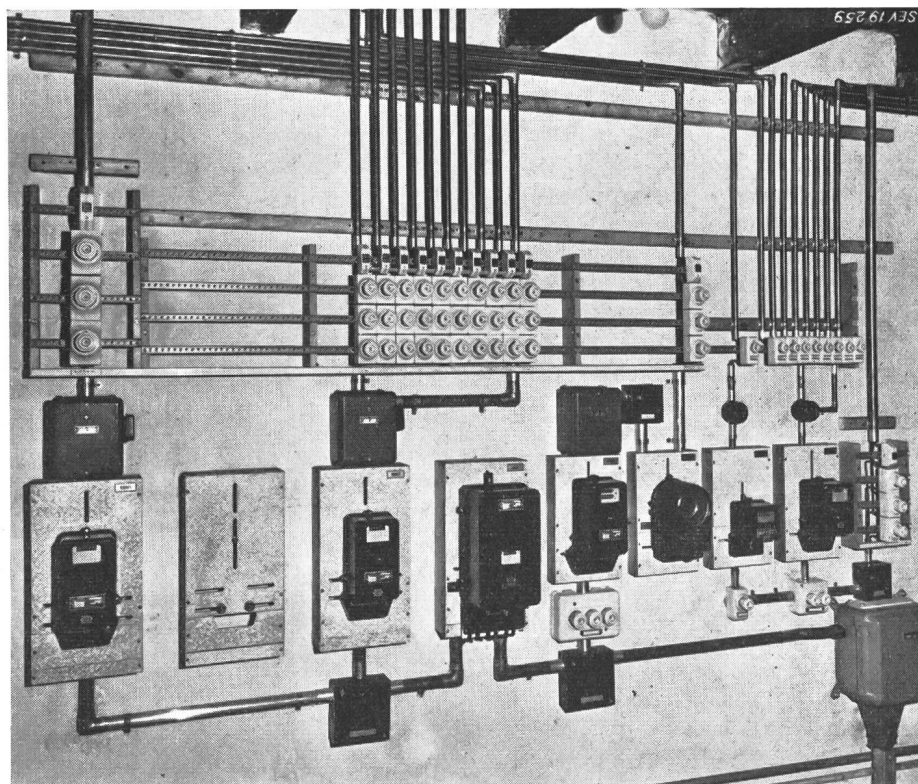
Fig. 47 Appareillage de distribution avec dispositifs de mesure pour entreprise commerciale Installé en 1951 selon la nouvelle méthode
