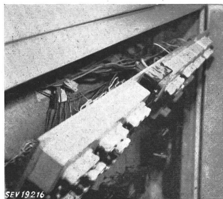
Fig. 6 Grand tableau de la fig. 5, en position ouverte Les connexions libres et mal disposées à l'arrière du tableau peuvent provoquer de grands dégâts
