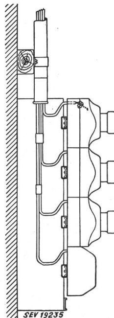
Fig. 23 Ligne conduite derrière des socles de coupe-circuit
