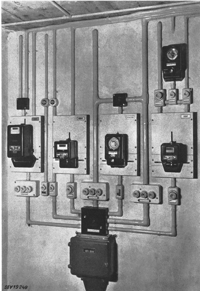
Fig. 27 Appareillage de distribution dans la cave d'un immeuble locatif Installé en 1951 Les coupe-circuit des dérivations sont situés aux divers étages
