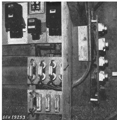
Fig. 42 Détails de l'installation de la fig. 41
