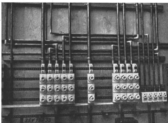
Fig. 21 Modèle d'appareillage de distribution et de protection, avec lignes sur deux plans différents Vue de devant
