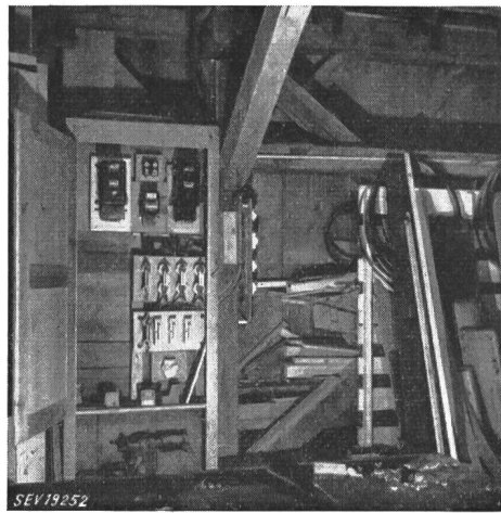
Fig. 41 Ancienne installation de coupe-circuit et de mesure d'une menuiserie
