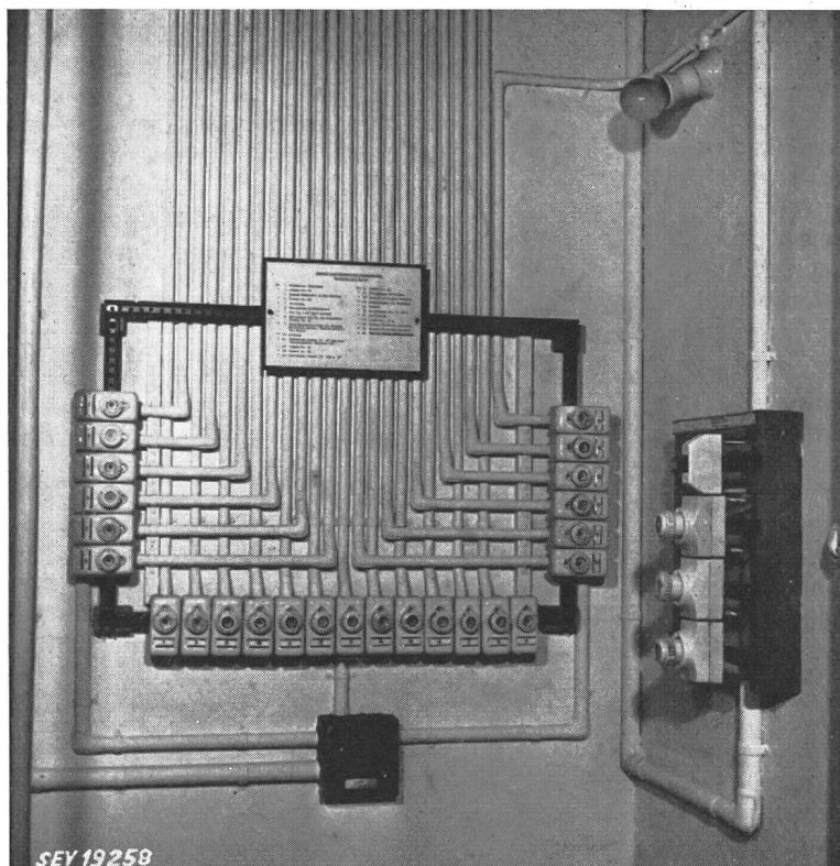
Fig. 46 Ancienne installation de distribution dans un emplacement très étroit, transformée en appliquant la nouvelle méthode de montage
