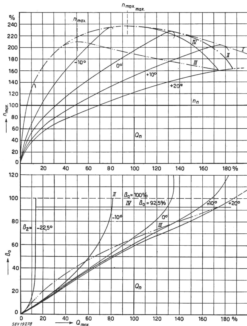
Fig. 2 Verlauf der Durchgangsdrehzahl n_{max} und der Turbinenöffnung \beta_0 über dem Wasserdurchlass Q_{max} für eine Kaplan-turbine, bei 4 verschiedenen Stellungen der Laufradschaufeln I Hüllkurve der n_{max} ; II Begrenzungskurve für \beta_0 = 100\% ; III n_{max} mit Steuerzusammenhang für günstigste Turbine; IV n_{max} bei gestörtem Steuerzusammenhang mit konstantem \beta_0 = 92,5\%
