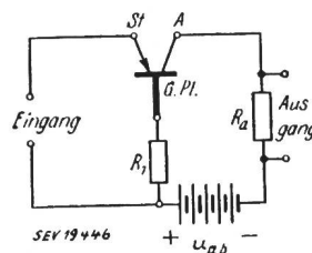
Fig. 3 Transistor-Gleichstromverstärker St Steuerspitze A Arbeitsspitze G.Pl. Grundplatte
