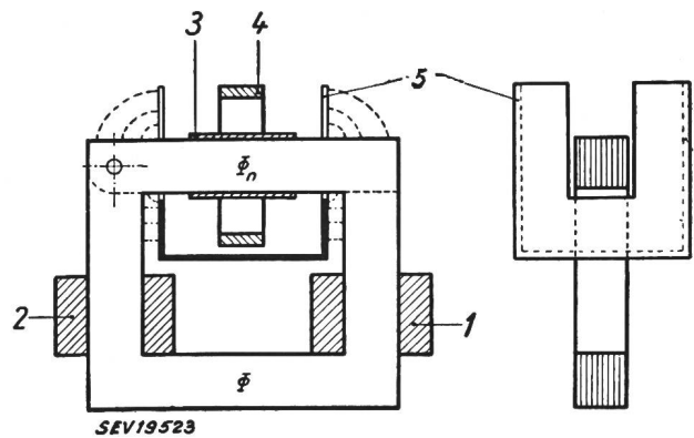
Fig. 1 Prinzip der Messung 1, 2 Erregerspulen; 3 Normalspule; 4 Prüfling; 5 Schirm
