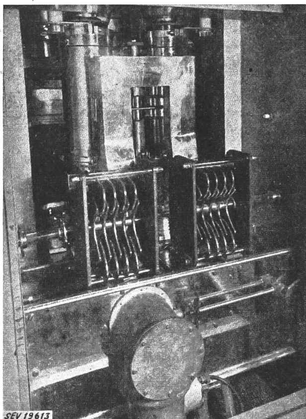
Fig. 4 Ansicht der End- und Auskoppelstufe des 45-kW-Bildsenders
