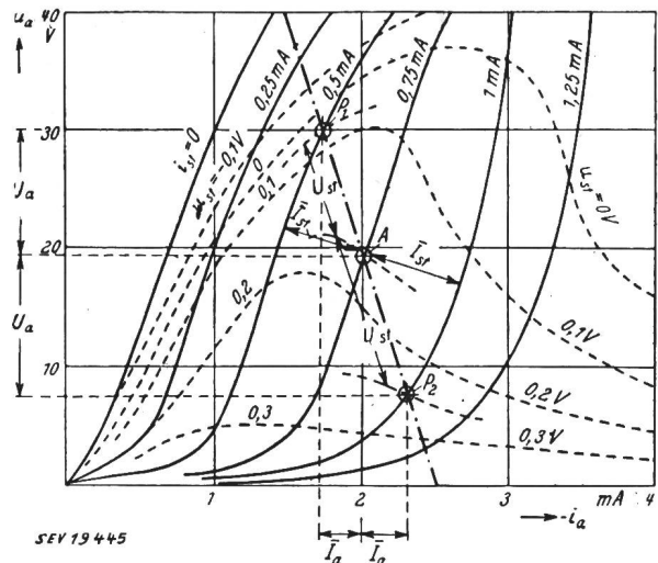
Fig. 2 Statisches u_a - i_a -Kennlinienfeld eines A-Transistors Erklärungen siehe im Text
