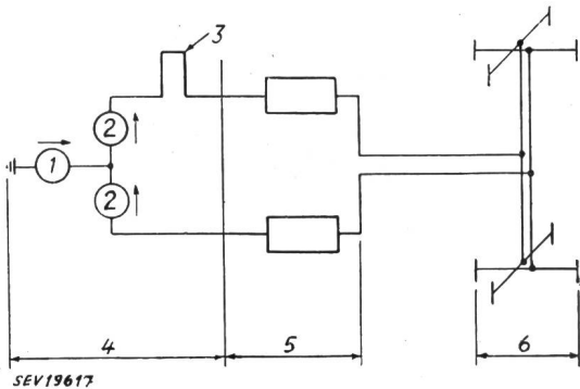
Fig. 8 Schema der Antennenanlage 1 Ton; 2 Bild; 3 90°-Schleife; 4 Diplexer; 5 Symmetrier-schleifen; 6 Antenne
