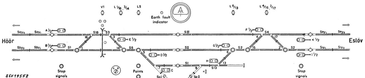
Fig. 2 Schema des Pult-Stellwerkes der Station Stehag
