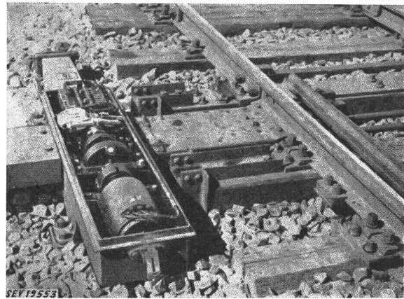
Fig. 1 Elektrischer Weichenantrieb
