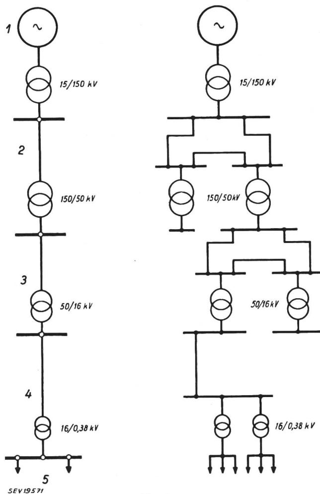
SEV 19571 Fig. 1 Schaltschemata von Energie-Übertragungssystemen 1 Stromerzeuger; 2 Hochspannungs-Übertragungsnetz; 3 Mittelspannungsnetz; 4 Hochspannungs-Verteilnetz; 5 Niederspannungs-Verteilnetz (Verbraucher)
