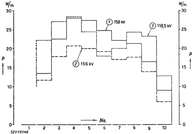
Fig. 10 Répartition longitudinale des pertes par effet de couronne. Tube de cuivre de 25 mm \phi 1 à sec, le matin du 7. 11. 51, sous 158 kV; 2 à sec, le soir, du 7. 11. 51, sous 156 kV; 3 sous pluie irrégulièrement répartie, le 16. 11. 51, sous 118,5 kV
