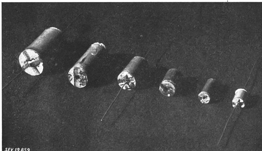
Fig. 5 Wickel aus Metallpapier mit Teilmetallisierung der Stirnseiten
