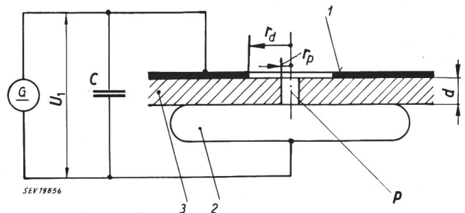
Fig. 2 Principalschema einer Anlage zur Untersuchung von Metallpapier
