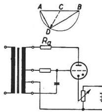
Steuerung des Zündeinsatzes einer Thyatronröhre
