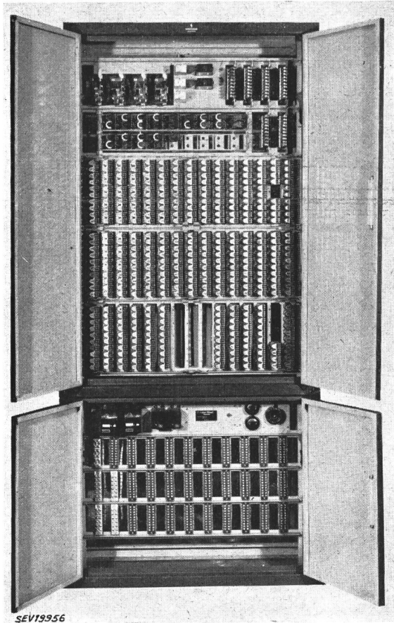
Fig. 2 Fernsteuer-Wählerapparat in Standschrank
