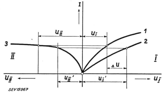
Fig. 6 Arbeitsdiagramm der beiden Ionisationskammern 1 Charakteristik der offenen Kammer ohne Rauch 2 Charakteristik der offenen Kammer mit Rauch 3 Charakteristik der geschlossenen Kammer
