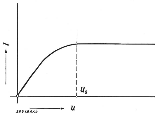
Fig. 3 Strom-Spannungscharakteristik einer Ionisationskammer U Spannung; U_s Sättigungsspannung; I Strom
