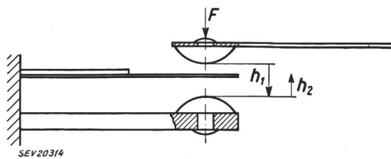
Fig. 3 Prellfreie Kontaktanordnung Bezeichnungen siehe im Text
