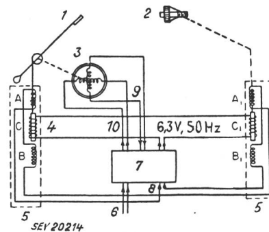
Fig. 3 Servomechanismus
