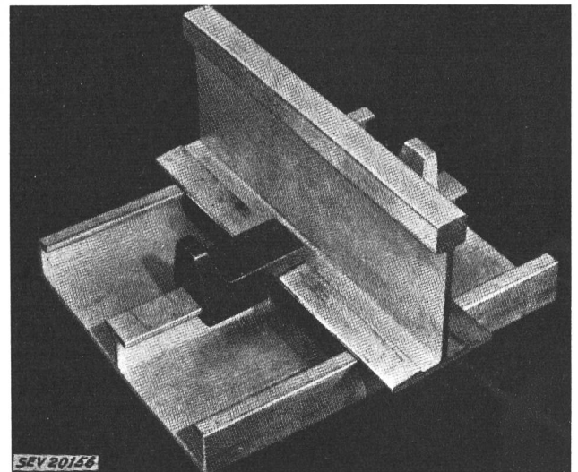
Fig. 2 Montagedetail
