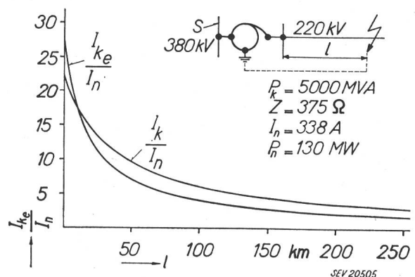
Fig. 2 Kurzschlußströme einer 220-kV-Leitung, angeschlossen über einen Transformator an ein 380-kV-System P_k Kurzschlussleistung; Z Wellenwiderstand; I_k Kurzschlussstrom; I_{ke} Erdschlussstrom; I_n Strom entspricht natürlicher Leistung; P_n natürliche Leistung; L Leitungslänge
