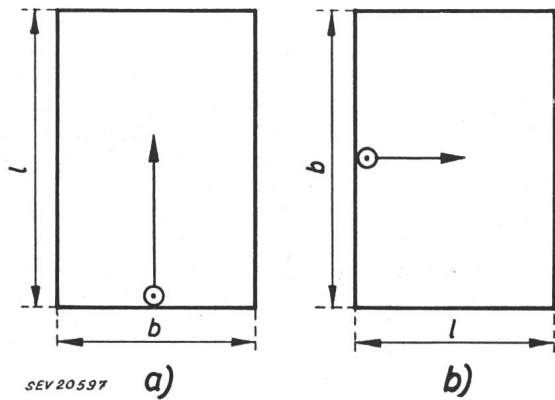
SEV 20597 a) b) Fig. 1 Raum-Grundriss, bezogen auf die Blickrichtung a und b geben an, in welcher Kolonne der Tabellen die betreffenden Raummasse aufzusuchen sind [Vgl. Fussnote 1) der Tabellen IIa...VIIa] © Beobachter; b Breite; l Länge Der Pfeil gibt die Blickrichtung an
