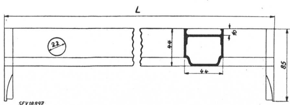
Bobine d'inductance avec enroulement antagoniste, dans un tube d'aluminium de profil spécial, qui porte deux douilles
