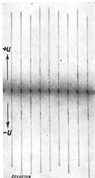
Fig. 9 Exemple d'un oscillogramme des tensions de contournement de l'isolateur de suspension représenté sur la fig. 1 9 chocs positifs et 9 chocs négatifs
