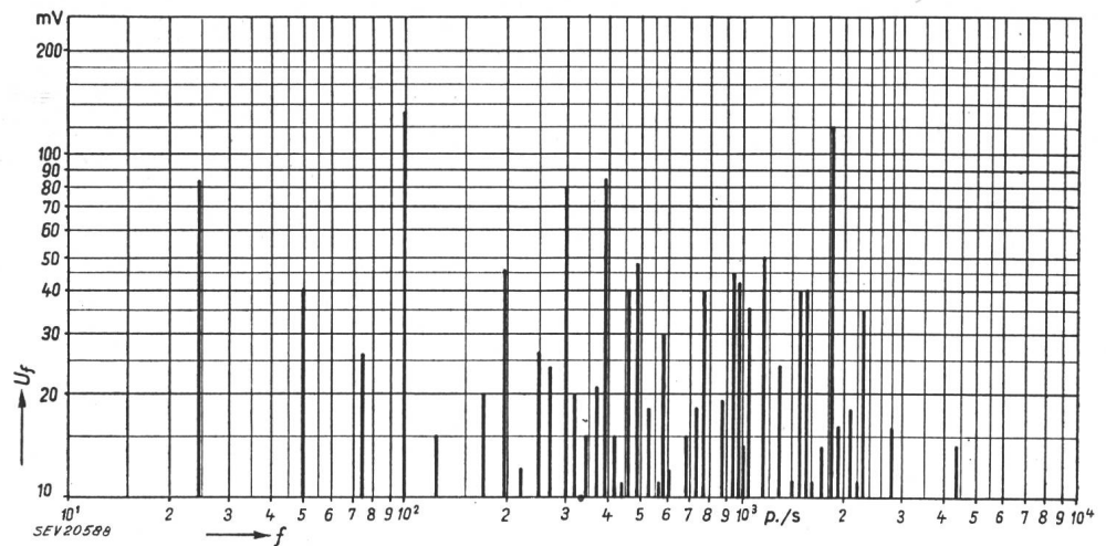
Fig. 5 Analyse de la tension d'une machine téléphonique à shunt magnétique U_n = 50 \text{ V} ; I = I_n = 400 \text{ A} ; env. 1500 t./min à vide U_f tension des harmoniques (valeur efficace)
