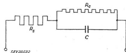
Fig. 9 Circuit équivalent du condensateur électrolytique C capacité; R_s résistance série; R_c résistance parallèle
