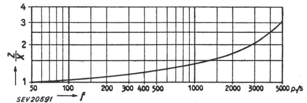
Fig. 8 Condensateur électrolytique STR Variation du rapport impédance/réactance ( Z/X ) en fonction de la fréquence f (cf. fig. 9)
