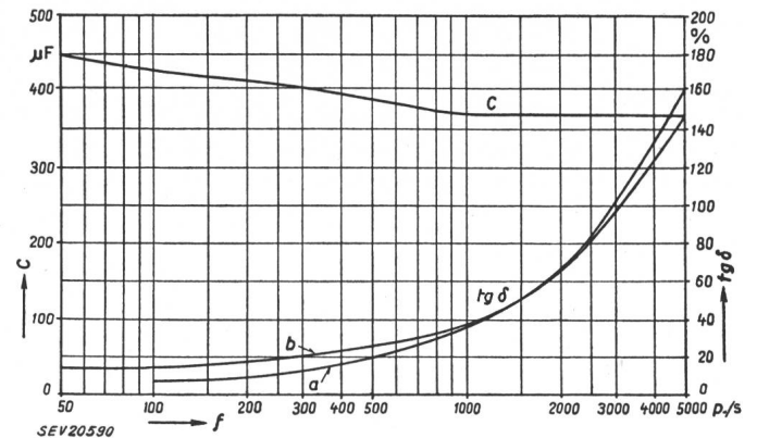
Fig. 7 Condensateur électrolytique STR Variation de la capacité C et de la tg \delta en fonction de la fréquence f
