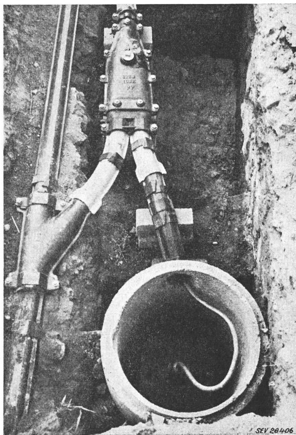
Fig. 1 Fernkabel mit Abzweigmuffe und Pupinschacht
