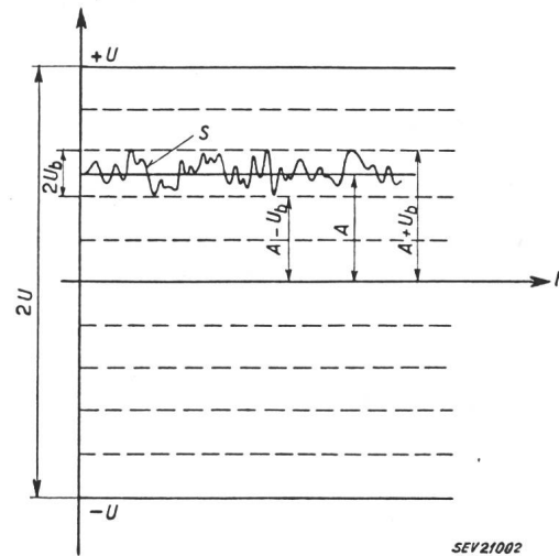
Fig. 2 Incertitude de la valeur instantanée du signal due au bruit S signal continu avec bruit A amplitude du signal continu sans bruit A + U_b amplitude maximum du signal avec bruit A - U_b amplitude minimum du signal avec bruit U_b amplitude maximum du bruit de puissance B U amplitude maximum du signal avec bruit de puissance totale P
