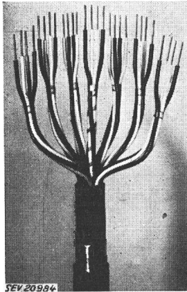
Fig. 11 Câble téléphonique à isolation polythène pour la transmission d'ondes porteuses (7x4x1,3 mm)
