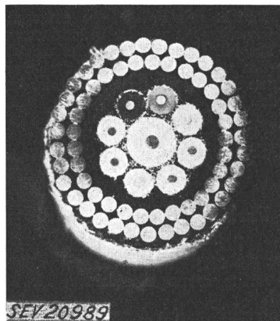
Fig. 17 Câble spécial à isolation polythène pour la station d'étude de la foudre au San Salvatore ( 1 \times 7 mm 2 + 8 \times 2,5 mm 2 ) Armure en cuivre mi-dur de 546 mm 2 de section
