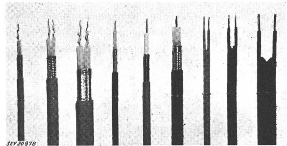
Fig. 5 Câbles d'antennes
