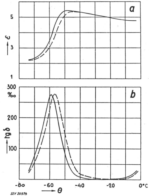
Fig. 2 Constante diélectrique ( \epsilon ) et angle de pertes ( \text{tg} \delta ) à basse température du plastifiant Di-2-éthyl-hexyl-phthalate ——— f = 800 \text{ Hz} ; - - - - f = 1600 \text{ Hz}
