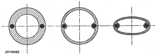
Fig. 10 Dessins schématiques de quelques exécutions de câbles tubulaires
