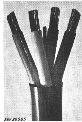
Fig. 12 Câble à basse tension à isolation et manteau en chlorure de polyvinyle (4x95 mm 2 )
