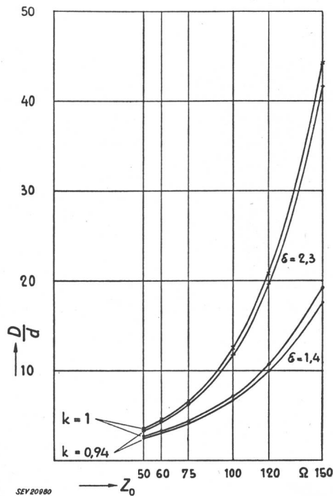
Fig. 7 Câbles coaxiaux
