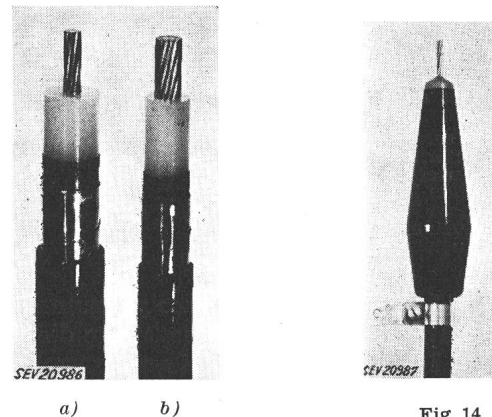
Fig. 13 Câble à haute tension à isolation polythène a 25 mm 2 — 20/11,5 kV b 50 mm 2 — 10/6 kV
