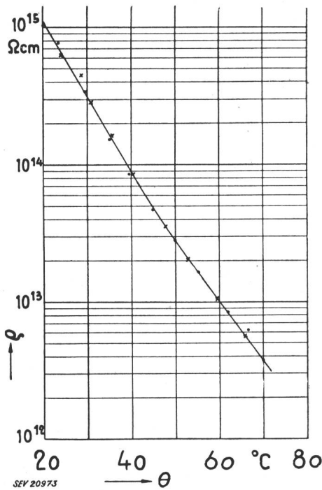
Fig. 1 Isolement en fonction de la température d'un PVC plastifié de haute résistivité \rho résistivité; \theta température
