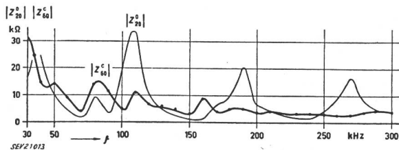
Fig. 6 Beträge der Leerlauf- und Kurzschlusswiderstände eines Starkstromtransformators 60/20 kV (Zweileiter-Kopplung) f Frequenz; Z Scheinwiderstand; Indizes: 0 Leerlauf; c Kurzschluss; 20 20-kV-Seite; 60 60-kV-Seite — |Z_{60}^o| Leerlaufwiderstand, 60-kV-Seite — |Z_{20}^c| Kurzschlusswiderstand, 20-kV-Seite
