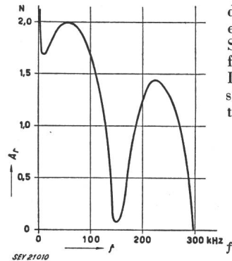
Fig. 3 Stossdämpfung einer Verbindung aus Freileitung, Kabel (0,5 km) und Sammelschienenleiter
