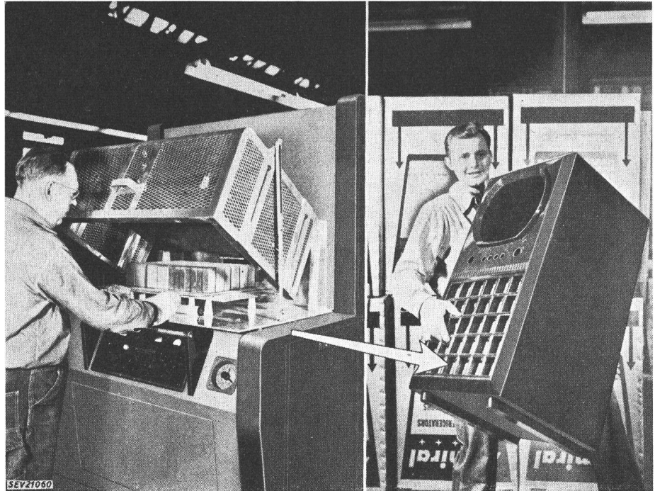
Fig. 10 Dielektrisches Vorwärmen von Kunststoffmasse vor dem Pressen von Fernsehempfängergehäusen
