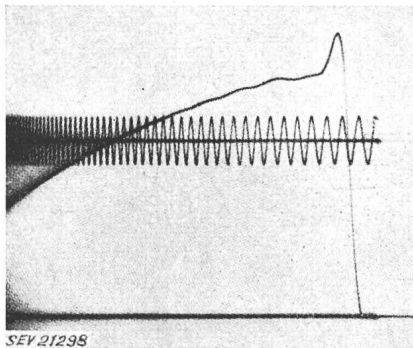
Fig. 3 Stoßspannung, registriert mit Universal-KO
