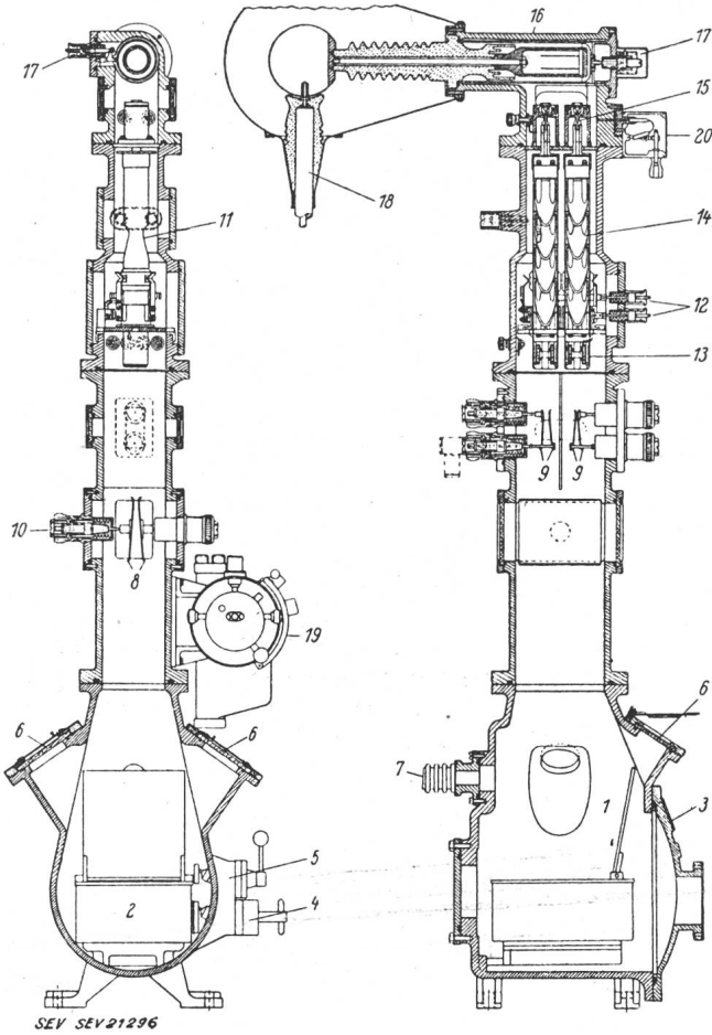
Fig. 1 2-Strahl-Hochspannungs-Kathodenstrahl-Oszillograph im Schnitt
