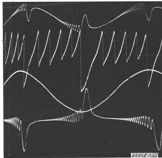
Fig. 4 Oszillogramm eines Vierstrahl-KO
