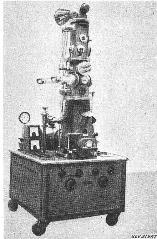
Fig. 2 4-Strahl-Hochspannungs-Oszillograph
