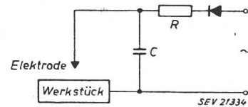
Grundschriftbild des Sparcatron-Verfahrens
