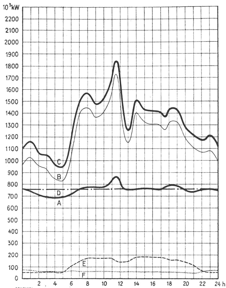
Diagramme de charge journalier du mercredi 14 octobre 1953
