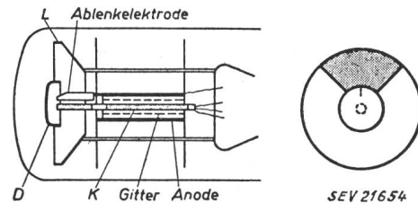
Fig. 1 Aufbau und Leuchtschirmbild des magischen Auges von Wagner D Abdeckkappe; K Kathode; L Leuchtschirm
