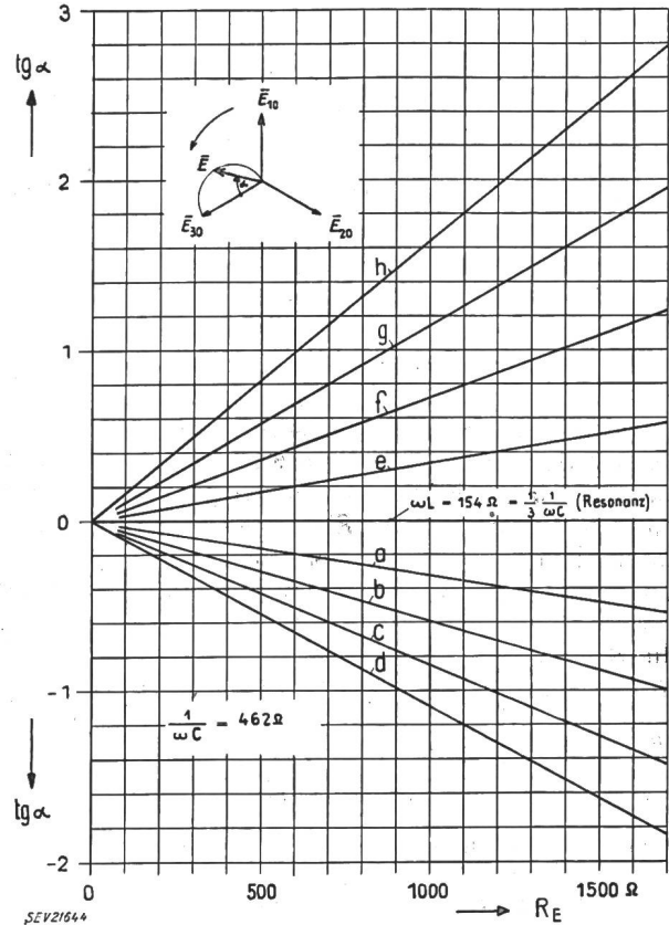
Fig. 4 \text{tg } \alpha in Funktion des Ohmschen Widerstandes an der Erdschlußstelle für verschiedene Einstellungen der Löschspule R_E Ohmscher Widerstand an der Erdschlußstelle
