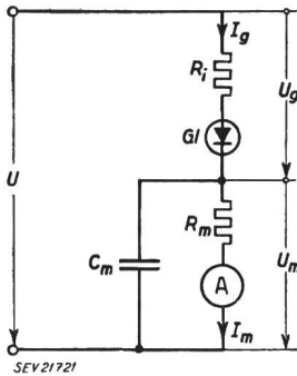
Fig. 1 Gleichrichterschaltung R_m C_m = T_m \gg T R_i Innenwiderstand des Gleichrichters GI R_m Innenwiderstand des Messinstrumentes A C_m Ladekondensator die zu messende Spannung U U_g Gleichrichterspannung U_m Messinstrumentenspannung I_g Gleichrichterstrom I_m Messinstrumentstrom T Periode der Spannungsimpulsfolge T_m Entladezeitkonstante
