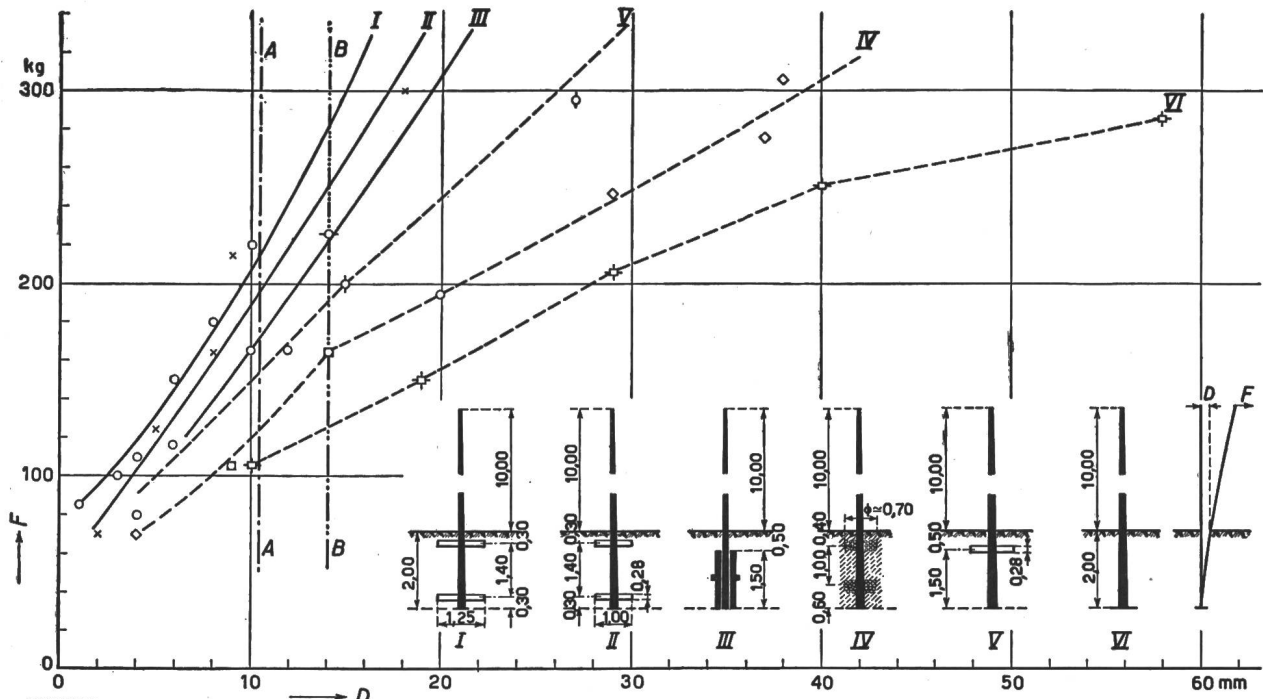
Fig. 1 Décollement en fonction de l'effort en tête pour différents types d'encastrement
