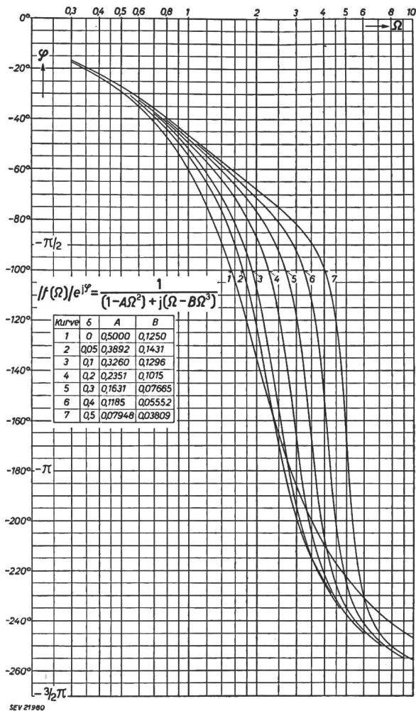
Blatt 5 Phasenmass der Spannungsübersetzung eines dreikreisigen Filters
