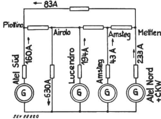
Fig. 2 Stromverteilung im Mitsystem
