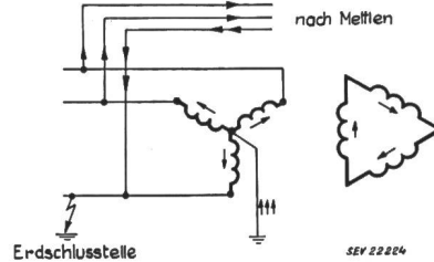
Fig. 6 Stromverteilung für Speisung durch das Kraftwerk
