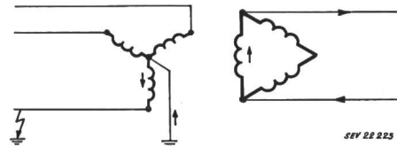
Fig. 6 Stromverteilung für Speisung durch das Kraftwerk
