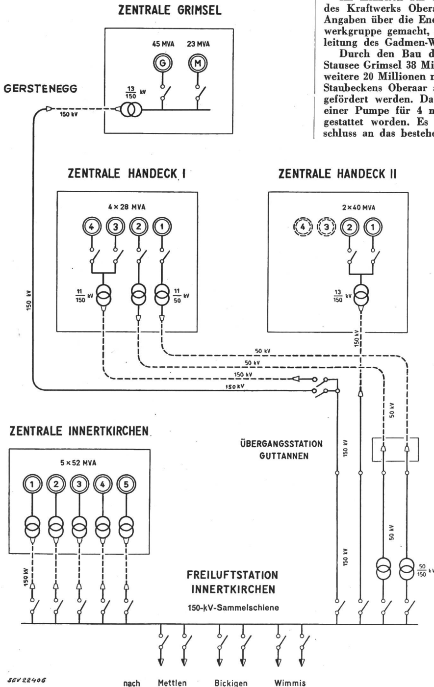
Fig. 4 Schema der Verbindung der Zentralen mit der Freiluftstation Innertkirchen G Turbinen-Generatorgruppe M Motor-Pumpengruppe 1...5 Turbinen-Generatorgruppen — Freileitung - - - - - Kabel
