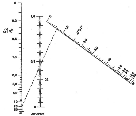
Fig. 5 Nomogramm zur Ermittlung der Hilfsgrösse \kappa
