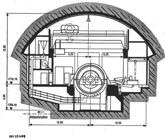
Fig. 8 Kraftwerk Grimsel Querschnitt C-C (vgl. Fig. 6)
