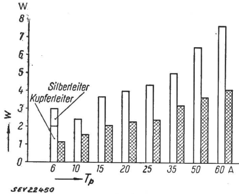
Fig. 7 Eigenverbrauch von Schmelzeinsätzen W Eigenverbrauch; T_p Typ nach Nennstromstärke □ Eigenverbrauch von flinken Schmelzeinsätzen und Belastung mit Nennstrom ▨ Eigenverbrauch von trägen Schmelzeinsätzen bei Belastung mit Nennstrom
