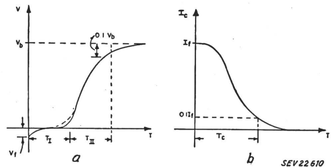
Fig. 2 Schaltzeiten in (a) Diode und (b) Transistor Bezeichnungen siehe im Text
